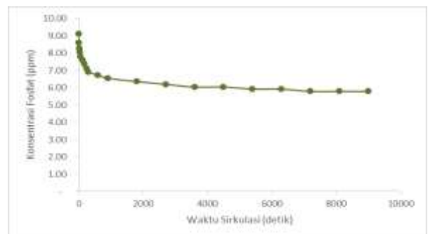
Gambar 5. Penurunan konsentrasi fosfat untuk penggunaan adsorbsi silika oksida 2 kg : karbon aktif 1 kg
